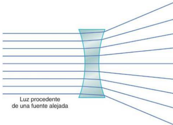
Figura 50-3. Desviación de los rayos luminosos en cada cara de una lente cóncava esférica, que muestra la divergencia de los rayos de luz paralelos.
