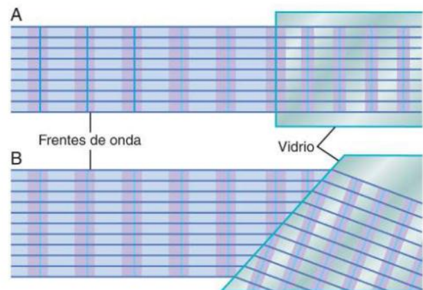
Figura 50-1. Rayos luminosos que penetran en una superficie de vidrio perpendicular a ellos ( A ) o que forme un ángulo con su trayectoria ( B ). Esta imagen pone de manifiesto que la distancia entre las ondas una vez que han entrado en el vidrio se acorta más o menos dos tercios con respecto al aire. También muestra que los rayos luminosos se desvían al chocar contra una superficie de vidrio que forme un ángulo.
