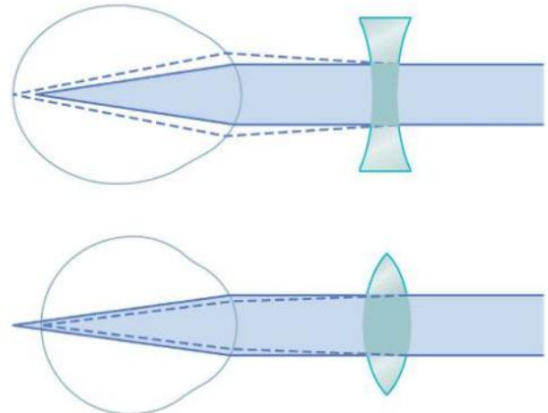
Figura 50-13. Corrección de la miopía con una lente cóncava (arriba) y de la hipermetropía con una lente convexa (abajo).
