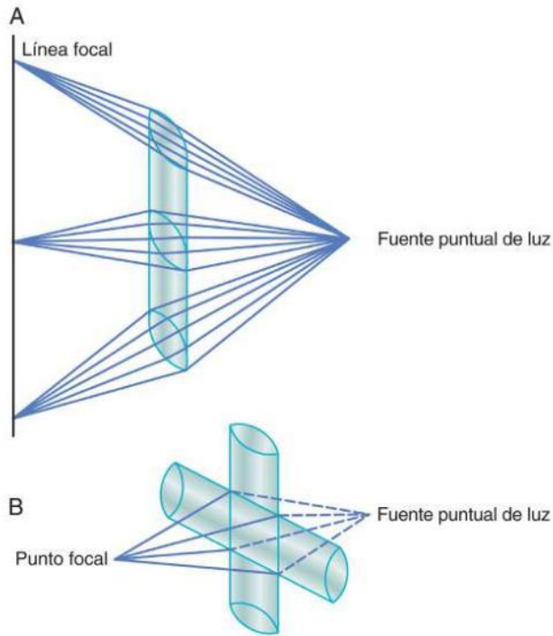
Figura 50-5. A. Concentración de la luz procedente de una fuente de partida en una línea focal mediante una lente cilíndrica. B. Dos lentes convexas cilíndricas que forman un ángulo recto entre sí, a fin de poner de manifiesto que una lente causa la convergencia de los rayos luminosos en un plano y la otra lo hace en el plano perpendicular a él. La combinación de ambas lentes proporciona el mismo punto focal que el obtenido con una sola lente convexa esférica.
